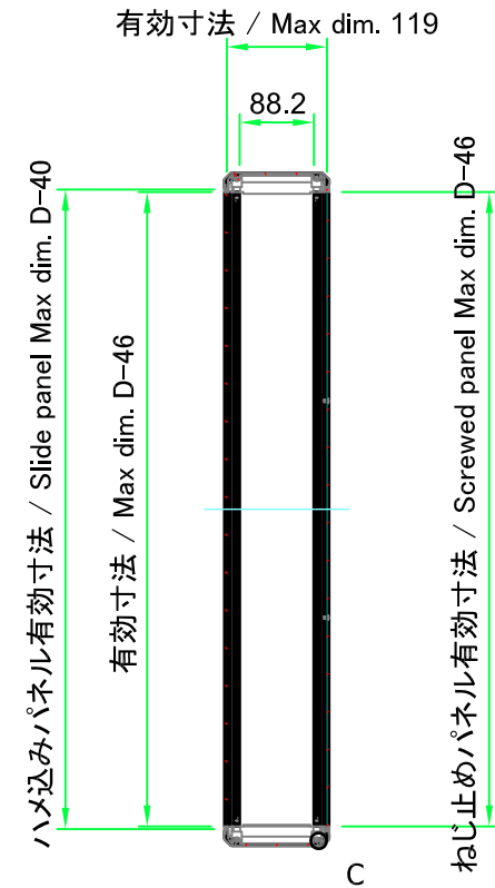
B-B ( 1 : 10 )
